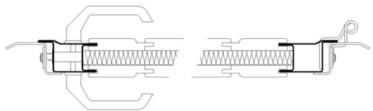
Abbildung zeigt Türe Pos.400 im Horizontalschnitt
